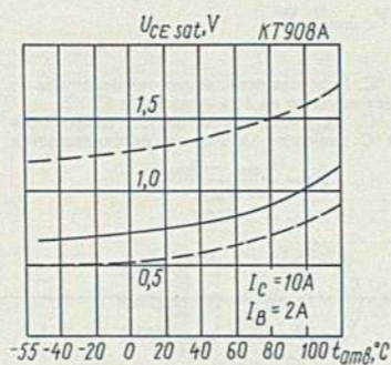
Зависимость напряжения насыщения коллектор-эмиттер от температуры окружающей среды Collector-emitter saturation voltage versus ambient temperature
