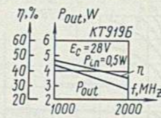
Зависимость выходной мощности и коэффициента полезного действия от частоты Output power and efficiency versus frequency
