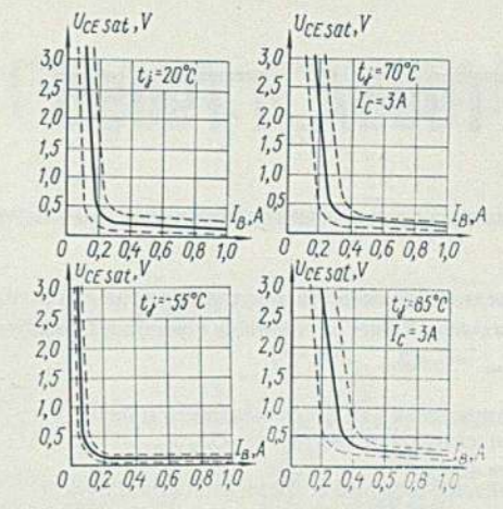
Зависимость напряжения насыщения коллектор-эмиттер от тока базы Collector-emitter saturation voltage versus base current
