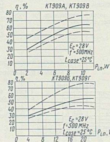
Зависимость коэффициента полезного действия от входной мощности
