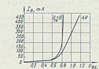
Типовые входные характеристики в схеме с общим эмиттером Standard input characteristics for common-emitter circuit
