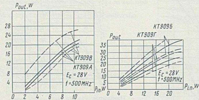
Зависимость выходной мощности от входной мощности
