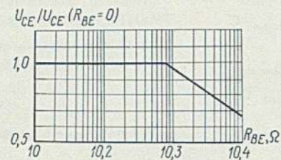
Зависимость относительной величины напряжения коллектор-эмиттер от сопротивления в цепи база-эмиттер Relative value of collector-emitter voltage versus resistance in base-emitter circuit
