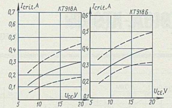
Зависимость критического тока коллектора от напряжения коллектор-эмиттер
