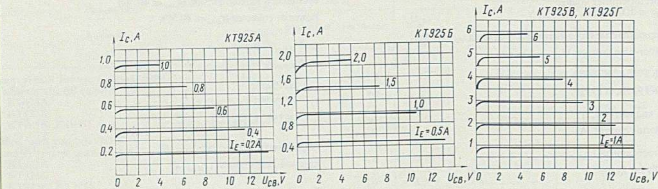
Типовые выходные характеристики в схеме с общей базой Standard output characteristics for common-base circuit
