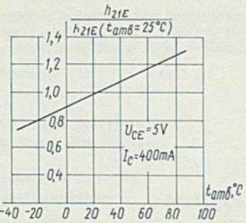
Зависимость относительной величины статического коэффициента передачи тока от температуры окружающей среды Relative value of static current-transfer ratio versus ambient temperature
