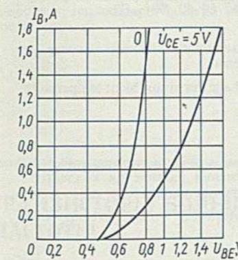
Типовые входные характеристики в схеме с общим эмиттером Standard input characteristics for common emitter circuit
