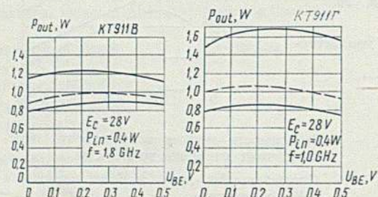
Зависимость выходной мощности от напряжения база-эмиттер Output power versus base-emitter voltage
