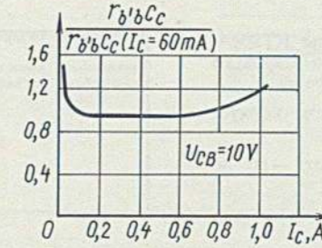
Зависимость относительной величины постоянной времени цепи обратной связи от тока коллектора Relative value of feedback circuit time constant versus collector current
