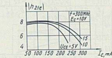
Зависимость модуля коэффициента передачи тока от тока коллектора Current-transfer ratio modulus versus collector current
