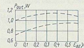
Зависимость выходной мощности от напряжения положительного смещения на базе Output power versus base positive bias
