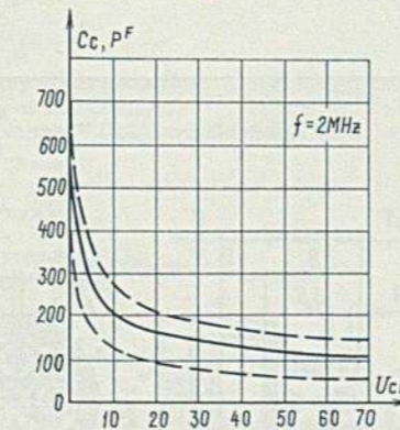
Зависимость емкости коллекторного перехода от напряжения коллектор-база Collector-junction capacitance versus collector-base voltage
