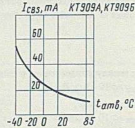
Зависимость начального тока коллектора от температуры окружающей среды
