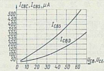
Зависимость обратного и начального тока коллектора от напряжения коллектор-база и коллектор-эмиттер Collector reverse and cut-off currents versus collector-base and collector-emitter voltages
