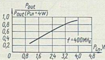
Зависимость относительной величины выходной мощности от входной мощности Relative value of output power versus input power
