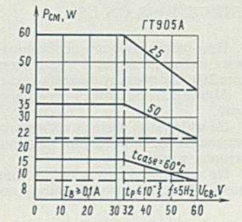
Зависимость наибольшей импульсной мощности на коллекторе от напряжения коллектор-база при различной температуре корпуса транзистора Maximum pulse power at collector versus collector-base voltage at various temperatures of transistor case
