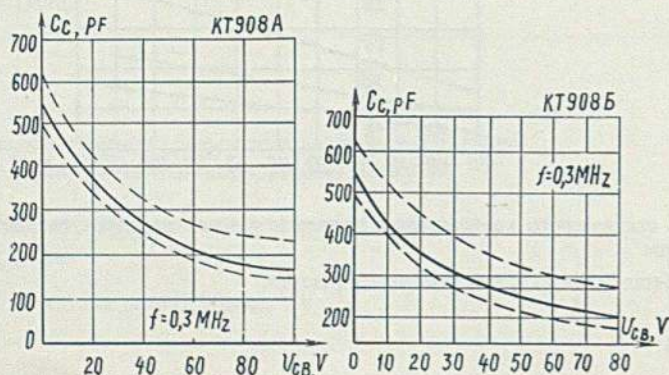
Зависимость емкости коллекторного перехода от напряжения коллектор-база Collector-junction capacitance versus collector-base voltage
