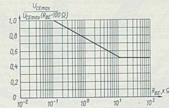
Зависимость относительной величины наибольшего напряжения коллектор-эмиттер от сопротивления в цепи база-эмиттер Relative value of maximum collector-emitter voltage versus resistance in base-emitter circuit
