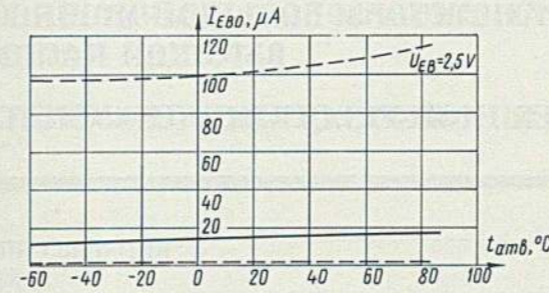
Зависимость обратного тока эмиттера от температуры окружающей среды
