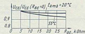
Зависимость относительной величины напряжения коллектор-эмиттер от сопротивления в цепи эмиттер-база
