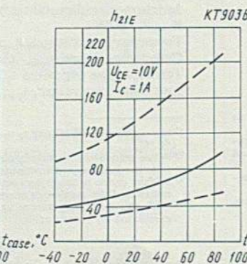
Зависимость статического коэффициента передачи тока от температуры корпуса Static current-transfer ratio versus case temperature
