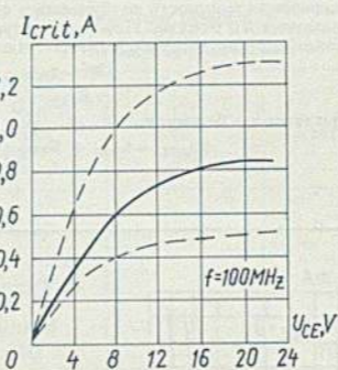
Зависимость критического тока от напряжения коллектор-эмиттер Critical current versus collector-emitter voltage
