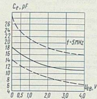
Зависимость емкости эмиттерного перехода от напряжения эмиттер-база Emitter-junction capacitance versus emitter-base voltage
