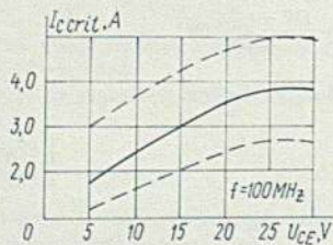
Зависимость критического тока коллектора от напряжения коллектор-эмиттер Collector critical current versus collector-emitter voltage
