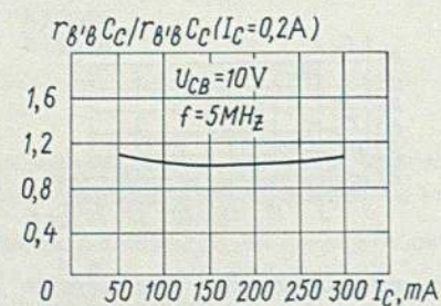
Зависимость относительной величины постоянной времени цепи обратной связи от тока коллектора Relative value of feedback circuit time constant versus collector current
