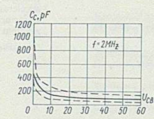
Зависимость емкости коллекторного перехода от напряжения коллектор-база Collector-junction capacitance versus collector-base voltage
