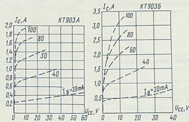
Типовые выходные характеристики в схеме с общим эмиттером (нижняя граница 95% разброса) Standard output characteristics for common-emitter circuit (lower boundary of 95% of spread)
