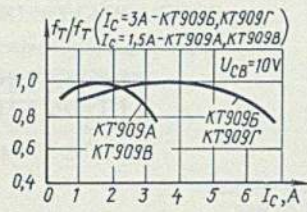
Зависимость относительной величины граничной частоты коэффициента передачи тока от тока коллектора
