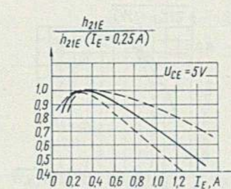
Зависимость относительной величины статического коэффициента передачи тока от тока эмиттера Relative value of static current-transfer ratio versus emitter current
