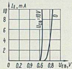
Входные характеристики в схеме с общей базой
