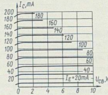
Выходные характеристики в схеме с общей базой
