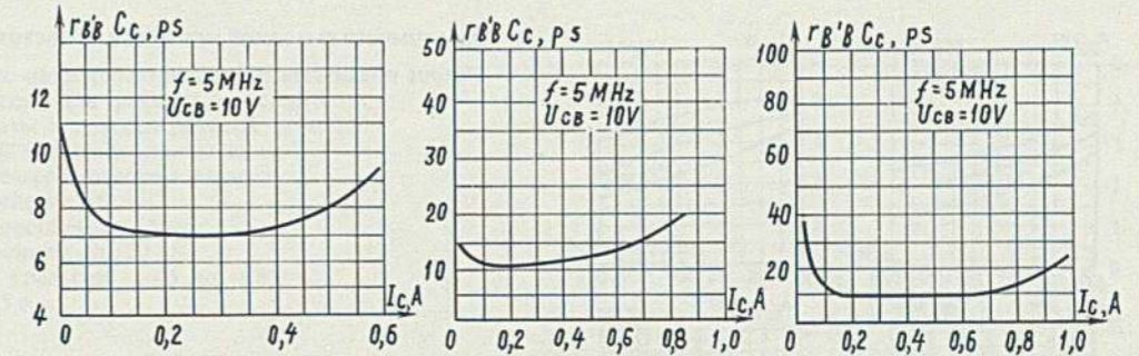
Зависимость постоянной времени цепи обратной связи от тока коллектора Feedback circuit time constant versus collector current
