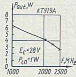
Зависимость выходной мощности от частоты Output power versus frequency
