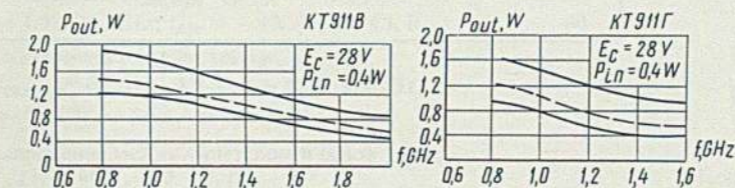
Зависимость выходной мощности от частоты Output power versus frequency
