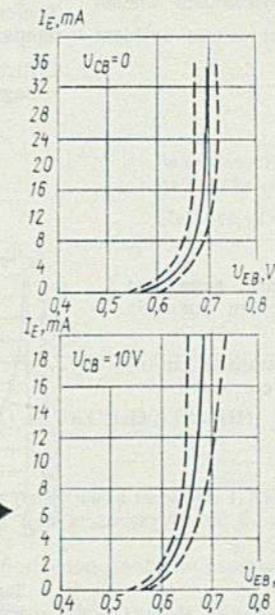
Типовая входная характеристика в схеме с общей базой Standard input characteristic for common-base circuit
