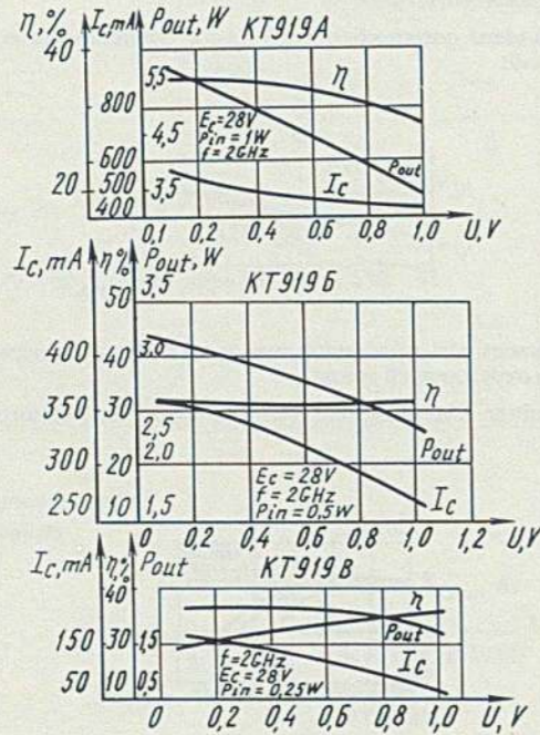
Зависимости выходной мощности, коэффициента полезного действия и тока коллектора от напряжения смещения Output power, efficiency and collector current versus bias
