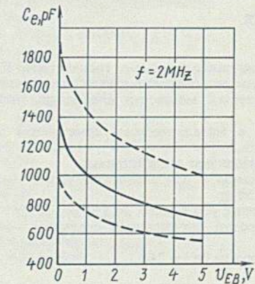
Зависимость емкости эмиттерного перехода от напряжения эмиттер-база Emitter-junction capacitance versus emitter-base voltage
