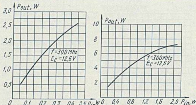
Зависимость выходной мощности от входной мощности
