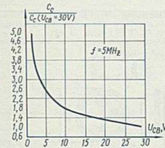
Зависимость относительной величины емкости коллекторного перехода от напряжения коллектор-база Relative value of collector-junction capacitance versus collector-base voltage
