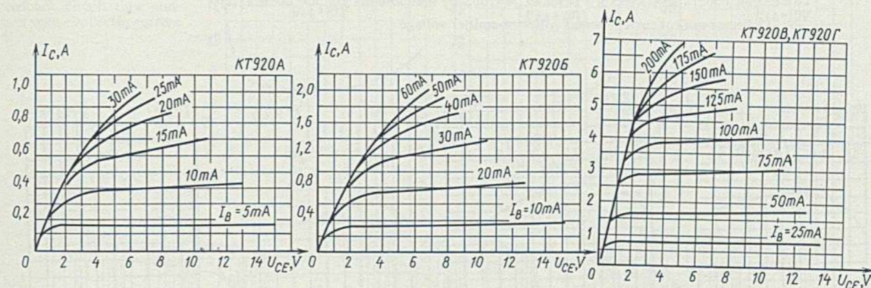
Типовые выходные характеристики в схеме с общим эмиттером Standard output characteristics for common-emitter circuit
