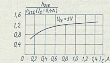
Зависимость относительной величины статического коэффициента передачи тока от тока коллектора Relative value of static current-transfer ratio versus collector current
