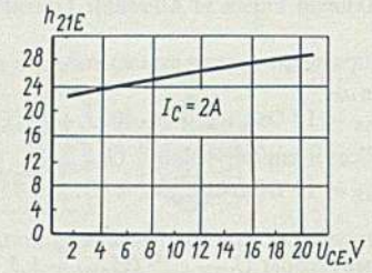
Зависимость статического коэффициента передачи тока от напряжения коллектор-эмиттер Static current-transfer ratio versus collector-emitter voltage
