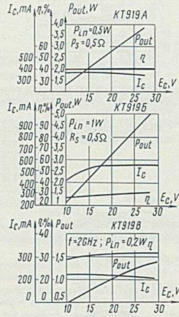
Зависимость выходной мощности, коэффициента полезного действия и тока коллектора от напряжения источника питания коллектора Output power, efficiency and collector current versus collector supply voltage
