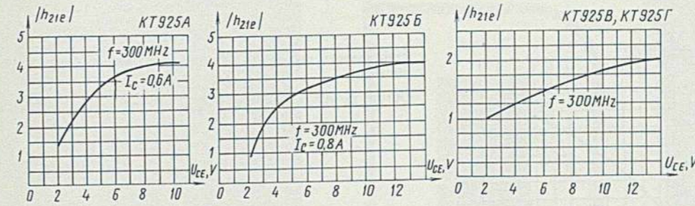
Зависимость модуля коэффициента передачи тока от напряжения коллектор-эмиттер Current-transfer ratio modulus versus collector-emitter voltage
