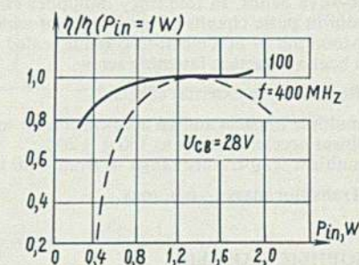
Зависимость относительной величины коэффициента полезного действия от входной мощности Relative value of efficiency versus input power
