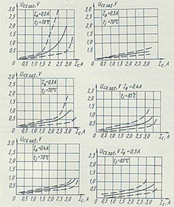
Зависимость напряжения насыщения коллектор-эмиттер от тока коллектора Collector-emitter saturation voltage versus collector current
