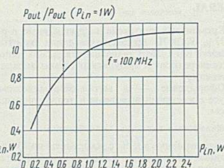
Зависимость относительной величины выходной мощности от входной мощности Relative value of output power versus input power
