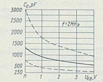
Зависимость емкости эмиттерного перехода от напряжения эмиттер-база Emitter-junction capacitance versus emitter-base voltage
