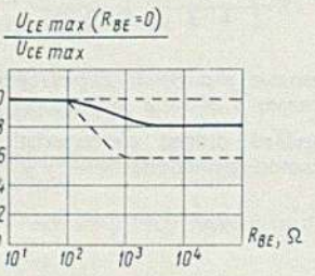
Зависимость относительной величины наибольшего напряжения коллектор-эмиттер от сопротивления в цепи база-эмиттер Relative value of maximum collector-emitter voltage versus resistance in base-emitter circuit
