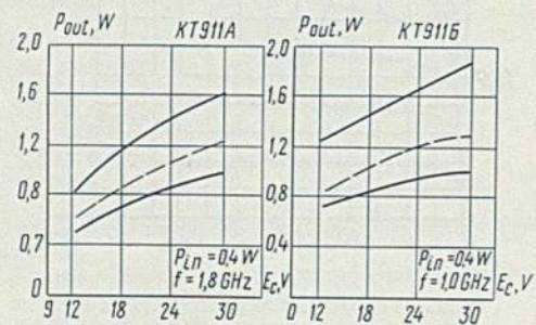
Зависимость выходной мощности от напряжения источника питания коллектора Output power versus collector supply voltage
