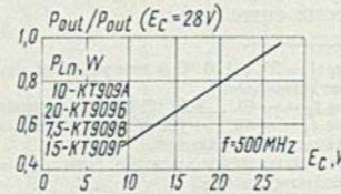
Зависимость относительной величины выходной мощности от напряжения источника питания коллектора
