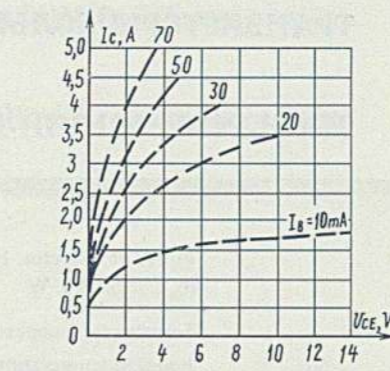
Верхние границы выходных характеристик в схеме с общим эмиттером
