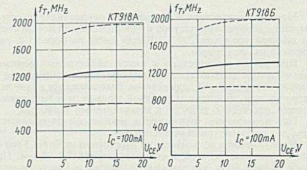
Зависимость граничной частоты коэффициента передачи тока от напряжения коллектор-эмиттер
