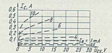
Нижние границы выходных характеристик в схеме с общим эмиттером Lower boundaries of output characteristics for common-emitter circuit
