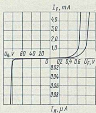
Вольтамперная характеристика диода Diode voltampere characteristic
