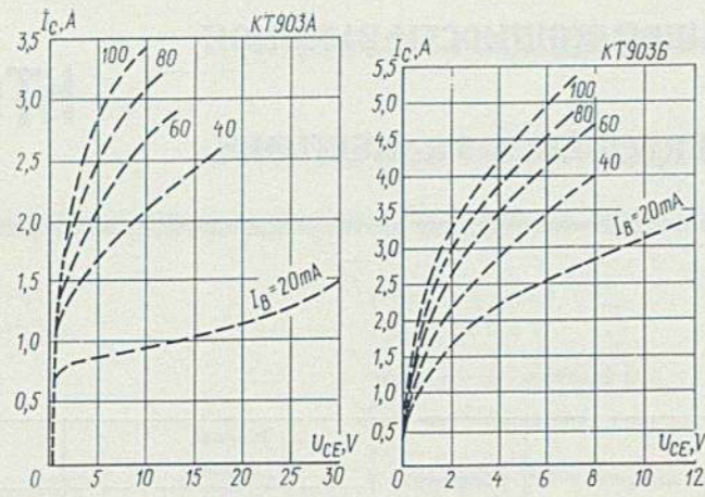
Типовые выходные характеристики в схеме с общим эмиттером (верхняя граница 95% разброса) Standard output characteristics for common-emitter circuit (upper boundary of 95% of spread)
