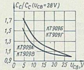
Зависимость относительной величины емкости коллекторного перехода от напряжения коллектор-база
