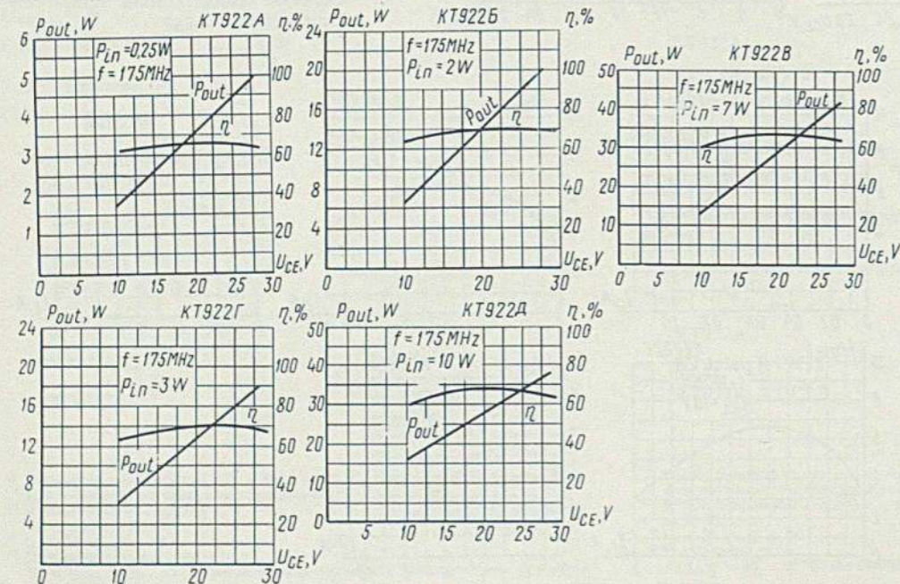
Зависимость выходной мощности и коэффициента полезного действия от напряжения коллектор-эмиттер Output power and efficiency versus collector-emitter voltage
