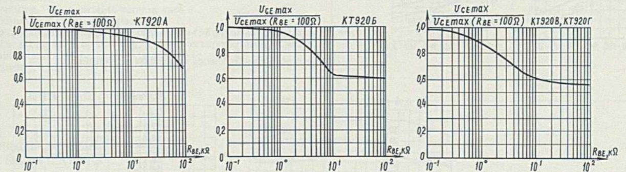
Зависимость относительной величины наибольшего напряжения коллектор эмиттер от сопротивления в цепи база-эмиттер Relative value of maximum collector-emitter voltage versus resistance in base-emitter circuit
