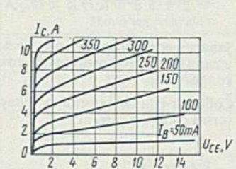
Типовые выходные характеристики в схеме с общим эмиттером Standard output characteristics for common-emitter circuit
