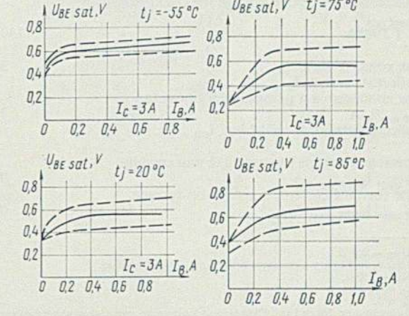
Зависимость напряжения насыщения база-эмиттер от тока базы Base-emitter saturation voltage versus base current
