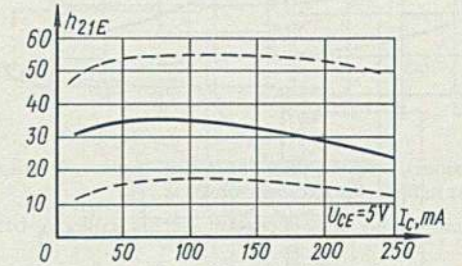
Зависимость статического коэффициента передачи тока в схеме с общим эмиттером от тока коллектора
