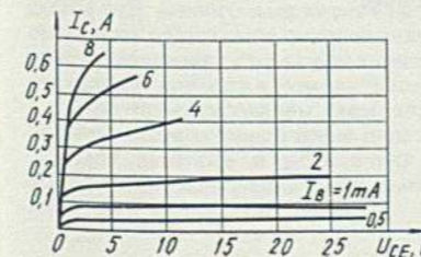
Типовые выходные характеристики в схеме с общим эмиттером Standard output characteristics for common-emitter circuit
