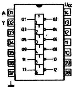
K155ЛН1
