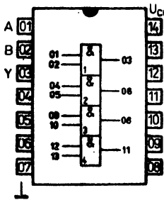
K155ЛИ1
