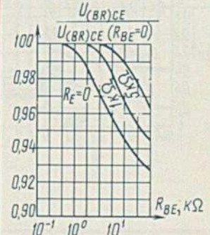
Зависимости относительной величины пробивного напряжения коллектор-эмиттер от сопротивления в цепи база-эмиттер
