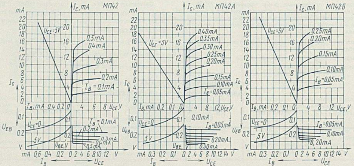
Статические характеристики в схеме с общим эмиттером
