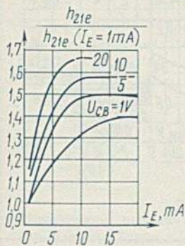
Зависимости относительной величины коэффициента передачи тока в режиме малого сигнала в схеме с общим эмиттером от тока эмиттера
