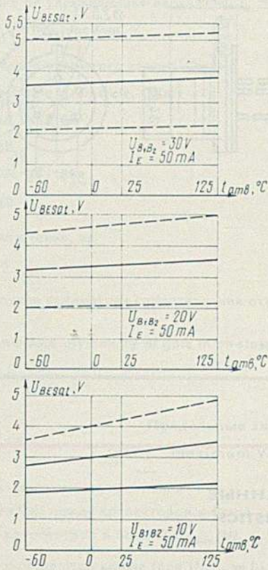
Зависимость остаточного напряжения от температуры окружающей среды
