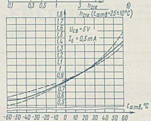
Зависимость относительной величины коэффициента передачи тока в схеме с общим эмиттером в режиме малого сигнала:
