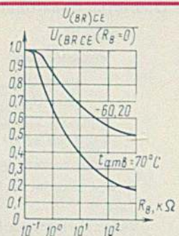
Зависимость относительной величины пробивного напряжения коллектор-эмиттер от сопротивления в цепи базы при различной температуре окружающей среды
