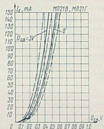
Входные характеристики в схеме с общей базой Input characteristics for common-base circuit
