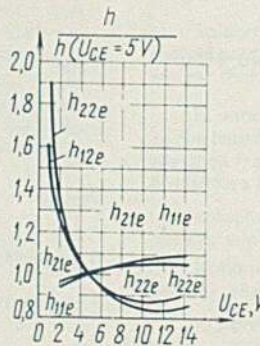
Зависимость относительного изменения h-параметров от напряжения коллектор-эмиттер
