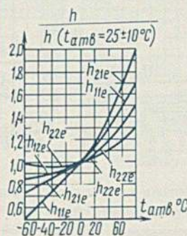
Зависимости относительной величины h-параметров от температуры окружающей среды
