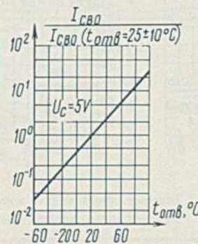
Зависимость относительной величины обратного тока коллектора от температуры окружающей среды
