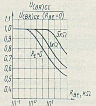
Зависимость относительной величины пробивного напряжения коллектор-эмиттер от сопротивления в цепи база-эмиттер
