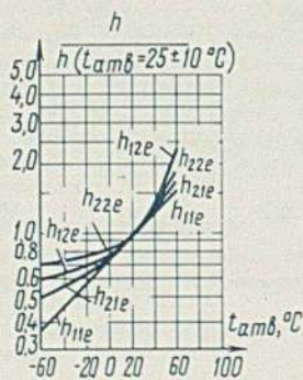
Зависимость относительного изменения h-параметров в схеме с общим эмиттером от температуры окружающей среды
