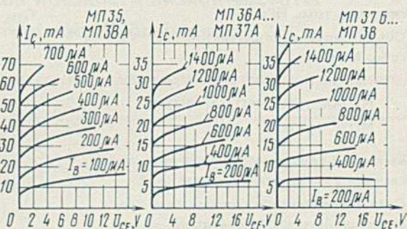
Типовые выходные характеристики в схеме с общим эмиттером
