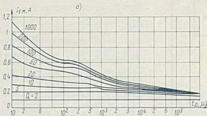
Зависимость импульсного тока эмиттера:
