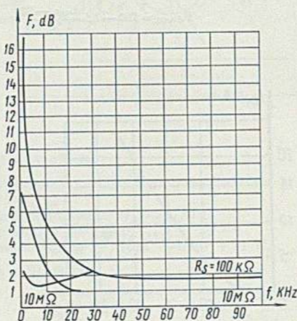
Зависимости коэффициента шума в зависимости от частоты при различном сопротивлении в цепи затвор-исток Noise factor versus frequency at various resistance in gate-source circuit
