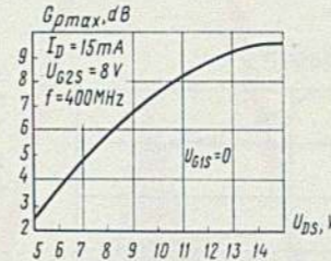
Типовая зависимость наибольшего коэффициента усиления по мощности напряжения сток-исток Standard relation between maximum power gain and drain-to-source voltage
