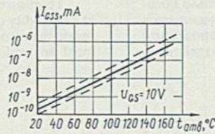
Зависимость тока затвора от температуры окружающей среды Gate current versus ambient temperature
