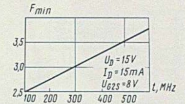
Типовая зависимость минимального коэффициента шума от частоты Standard relation between minimum noise factor and frequency
