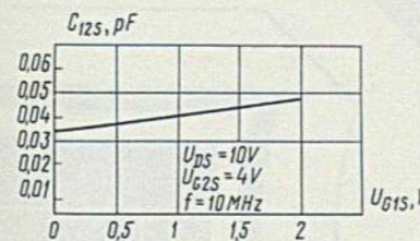
Типовая зависимость проходной емкости от напряжения затвор 1-исток Standard relation between transfer capacitance and 1-st gate-to-source voltage
