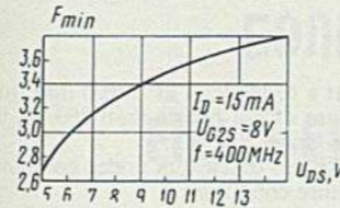
Типовая зависимость минимального коэффициента шума от напряжения сток-исток Standard relation between minimum noise factor and drain-to-source voltage
