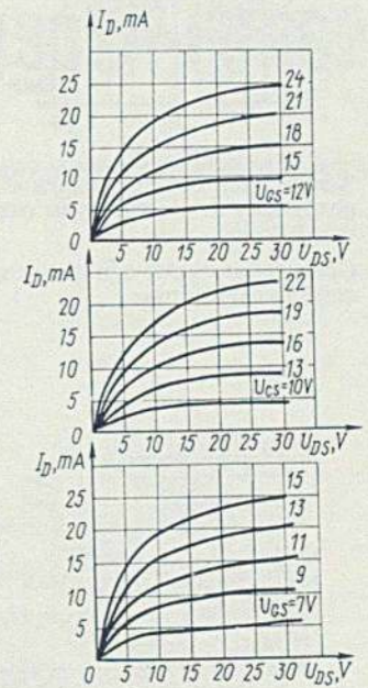
Входные характеристики при различных напряжениях затвор-исток Input characteristics at various gate-to-source voltages
