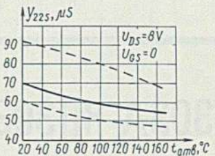
Зависимость полной выходной проводимости от температуры окружающей среды Open-circuit output admittance versus ambient temperature
