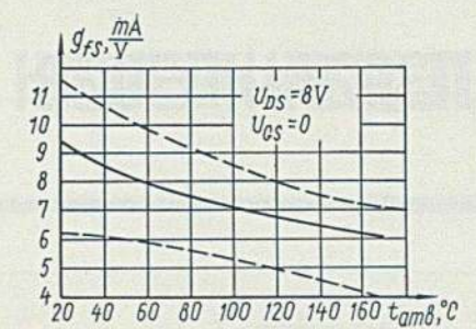
Зависимость крутизны характеристики от температуры окружающей среды Transconductance versus ambient temperature
