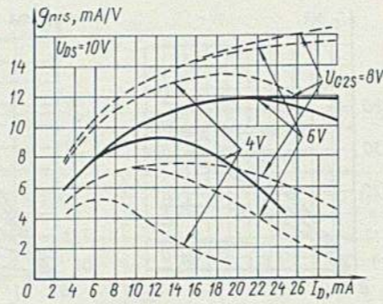
Зависимости крутизны характеристики от тока стока при различных напряжениях затвор 2-исток Transconductance versus drain current at various 2-nd gate-to-source voltages
