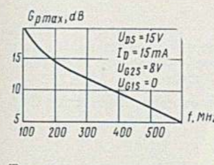
Типовая зависимость наибольшего коэффициента усиления по мощности от частоты Standard relation between maximum power gain and frequency
