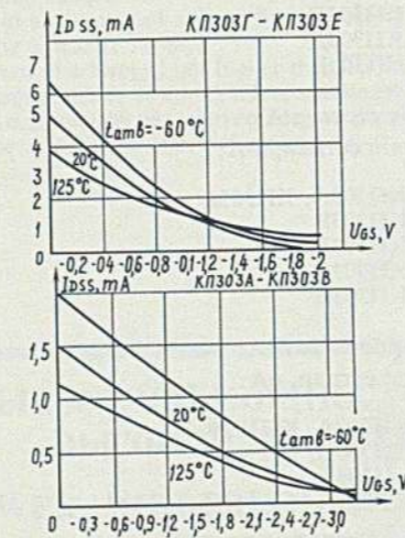
Зависимость тока стока от напряжения затвор-исток при различной температуре окружающей среды
