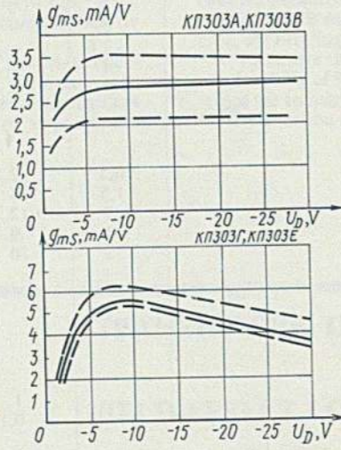
Зависимость крутизны характеристики от напряжения стока
