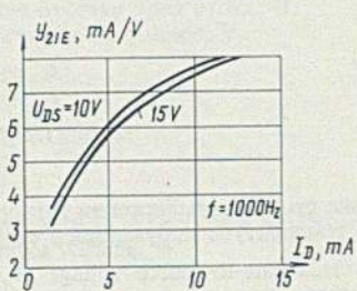
Типовая зависимость крутизны характеристики от тока стока Standard relation between transconductance and drain current
