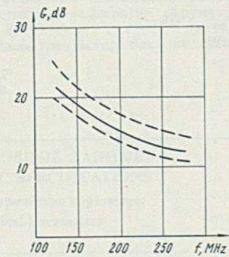
Зависимость коэффициента усиления по мощности от частоты Power gain versus frequency
