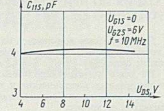
Типовая зависимость входной емкости от напряжения сток-исток Standard relation between input capacitance and drain-to-source voltage
