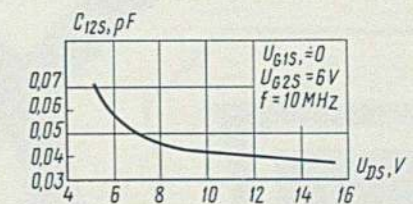
Зависимость проходной емкости от напряжения сток-исток Transfer capacitance versus drain-to-source voltage
