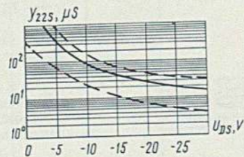
Зависимость полной выходной проводимости от напряжения сток-исток Open-circuit output admittance versus drain-to-source voltage
