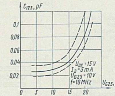
Зависимость проходной емкости затвор 1-исток от напряжения затвор 2-исток 1-st gate-source transfer capacitance versus 2-nd gate-to-source voltage
