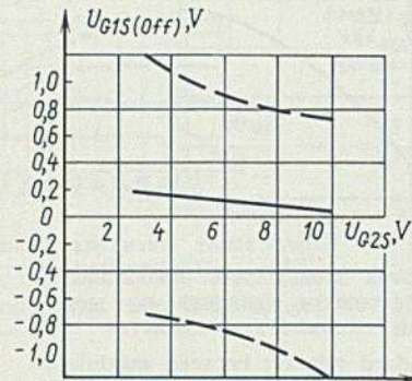
Зависимость напряжения отсечки по первому затвору от напряжения затвор 2-исток 1-st gate cut-off voltage versus 2-nd gate-to-source voltage
