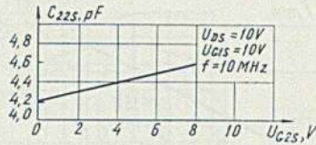
Типовая зависимость выходной емкости от напряжения затвор 2-исток Standard relation between output capacitance and 2-nd gate-to-source voltage
