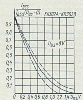
Зависимость относительной величины тока стока от напряжения затвор-исток Relative value of drain current versus gate-to-source voltage
