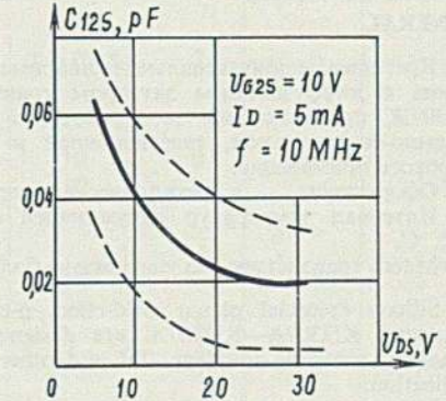
Зависимость проходной емкости затвор 1-сток от напряжения сток-исток 1-st gate-drain transfer capacitance versus drain-to-source voltage
