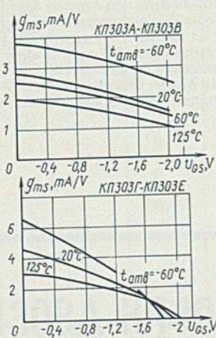
Зависимость крутизны характеристики от напряжения затвор-исток при различной температуре окружающей среды
