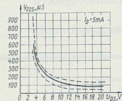
Зависимость полной выходной проводимости от напряжения сток-исток Open-circuit output admittance versus drain-to-source voltage
