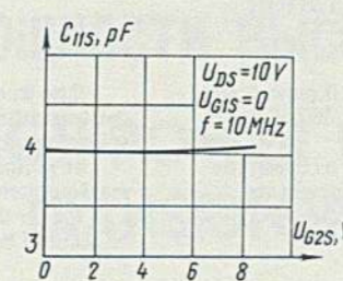
Типовая зависимость входной емкости от напряжения затвор 2-исток Standard relation between input capacitance and 2-nd gate-to-source voltage
